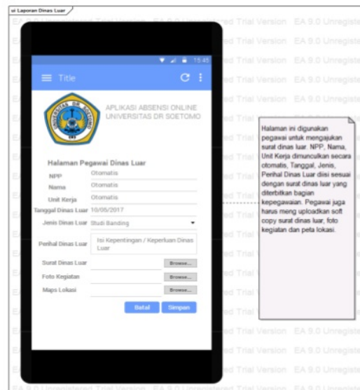
Gambar 4. GUI Dinas Luar Dosen dan tenaga kependidikan
