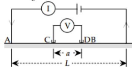
Gambar 4. Skema VES konfigurasi Schlumberger (Lowrie, 2007).
