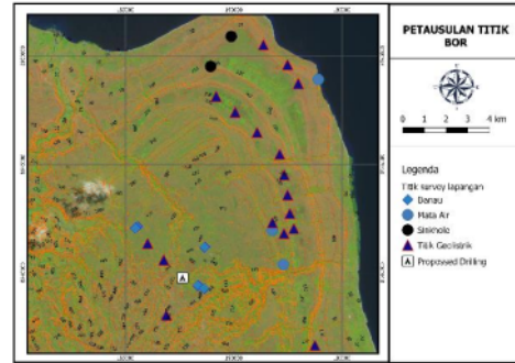
Gambar 12. Lokasi usulan titik bor
