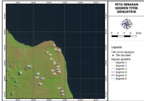
Gambar 11. Sebaran segmen lintasan geolistrik
