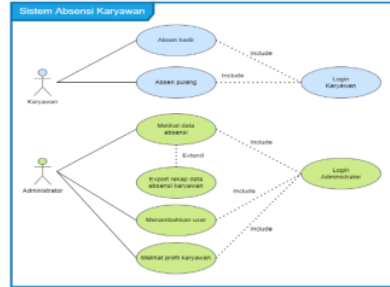
Gambar 4. Usecase Diagram Sistem Absensi Karyawan
