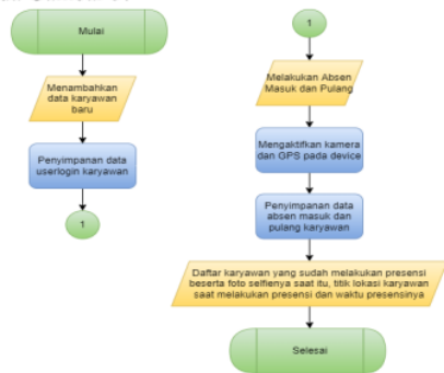
Gambar 3. Flowchart Sistem Absensi Karyawan
