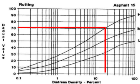
Grafik 1. Hubungan density dan deduct value untuk jenis kerusakan retak kulit buaya STA 0+000 s/d 0+200
