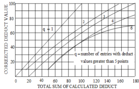
(Sumber : Shanin, Army Corp of Engineers USA 1994) Gambar 1. Grafik hubungan CDV dan TDV
