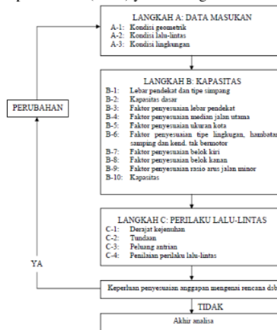
Gambar 4. Bagan Alir Perhitungan Kinerja Simpang Tak Bersinyal
