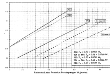
Gambar 5. Faktor Penyesuaian Lebar Pendekat ( F_w )
