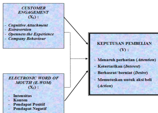
Gambar 2: Kerangka Konseptual
