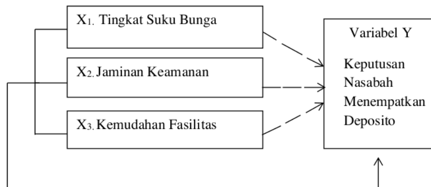
Gambar 1. Kerangka Konsep
