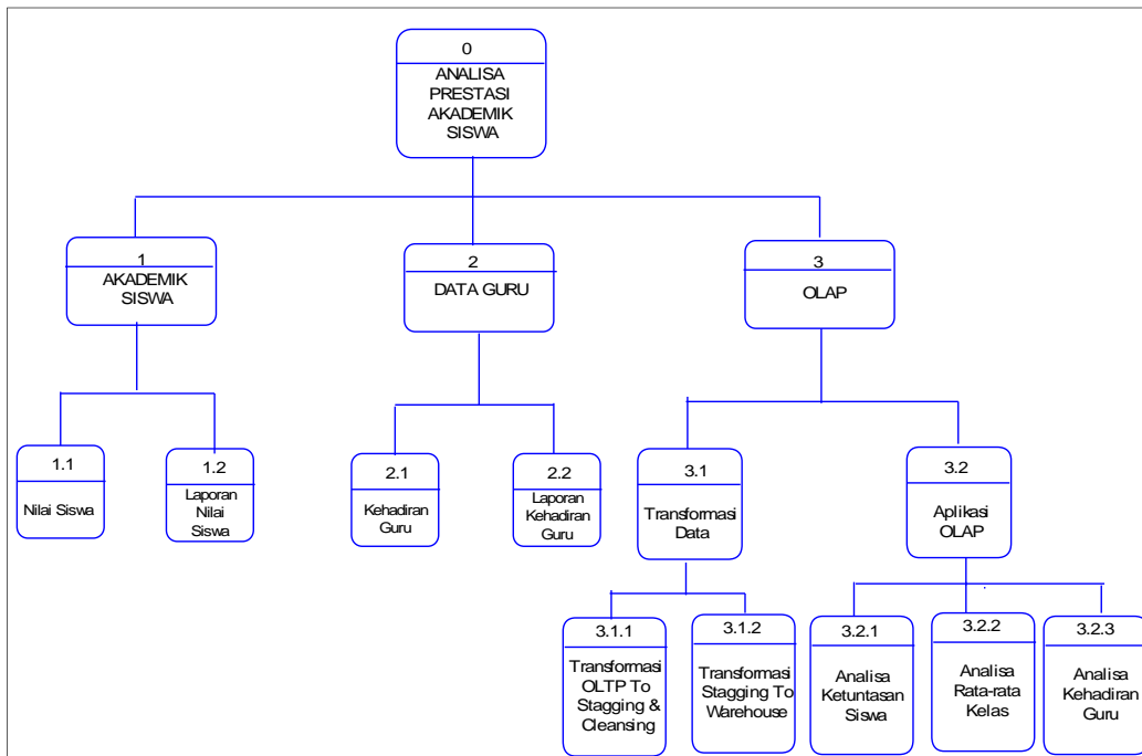
Gambar 6: Diagram Berjenjang
