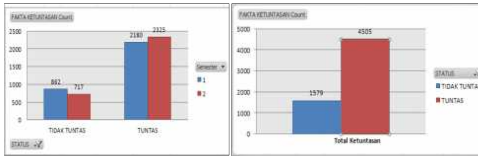
Gambar 12: Ketuntasan Siswa
